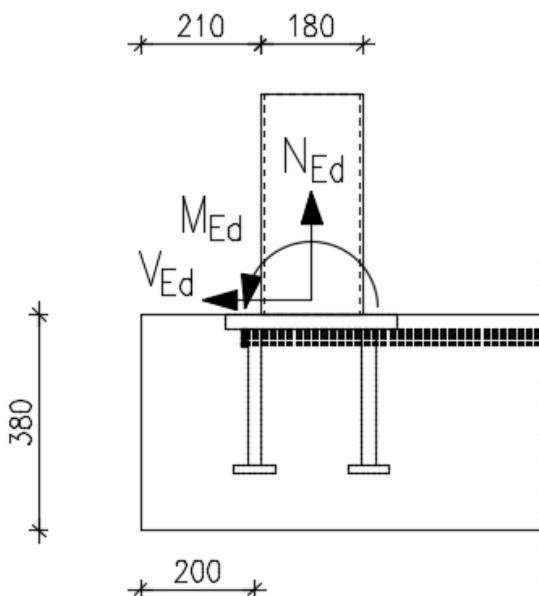
Kuva 9. Leikkausvoiman lisäraudoituksen sijoitus mitoitusesimerkissä
