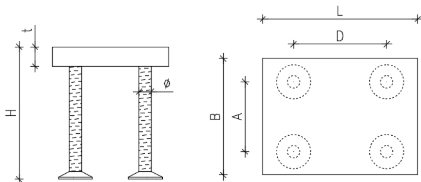
Kuva 1. JKL-kiinnityslevyjen mittojen merkinnät
